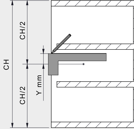
Simetrik İki Raf Uygulaması Symmetric Double Shelf Application
