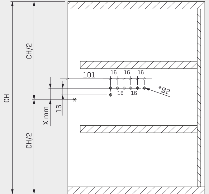
*Euro Vida kullanılıyorsa delikler Ø5mm olarak delinmelidir. *For usage of Euro Screw, the diameter of holes must be Ø5 mm.
