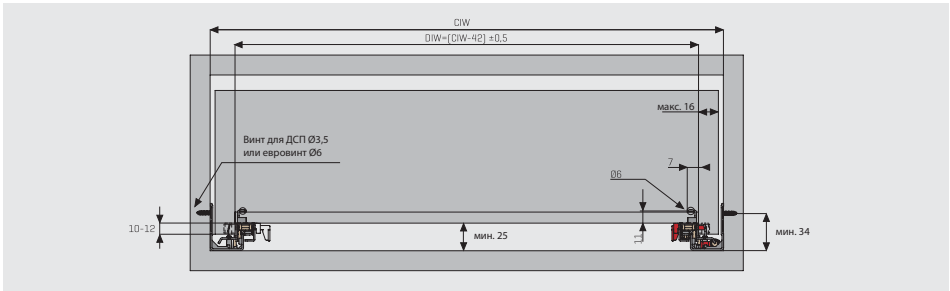
Расположение отверстий для направляющих Lock-Fix
