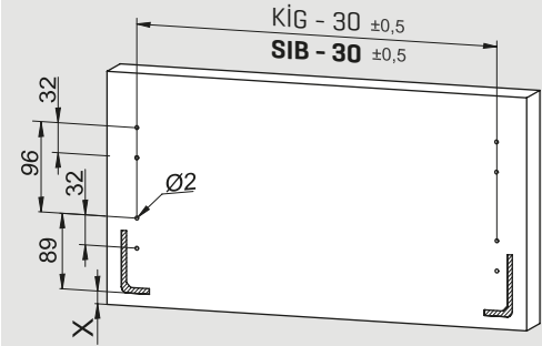
Ön Panel / Frontblende
